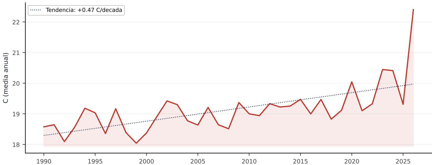
Temperatura media anual — ERA5-Land (nivel departamental: Tarija)
