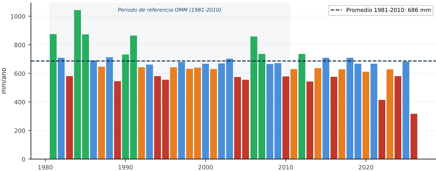
Precipitacion anual — CHIRPS v2.0 (nivel departamental: Tarija)
