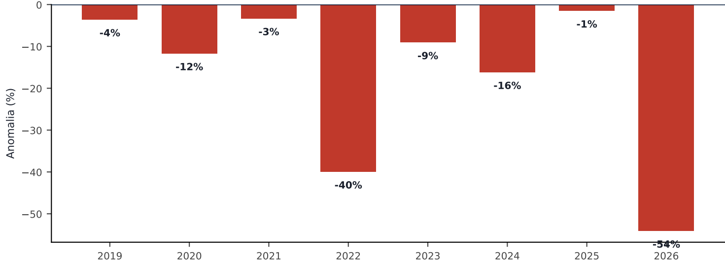
Anomalia de precipitacion vs. promedio 1981-2010 (%)
